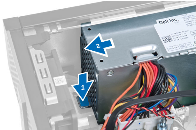
7. הרם את ספק הכוח והוצא אותו מהמחשב.
